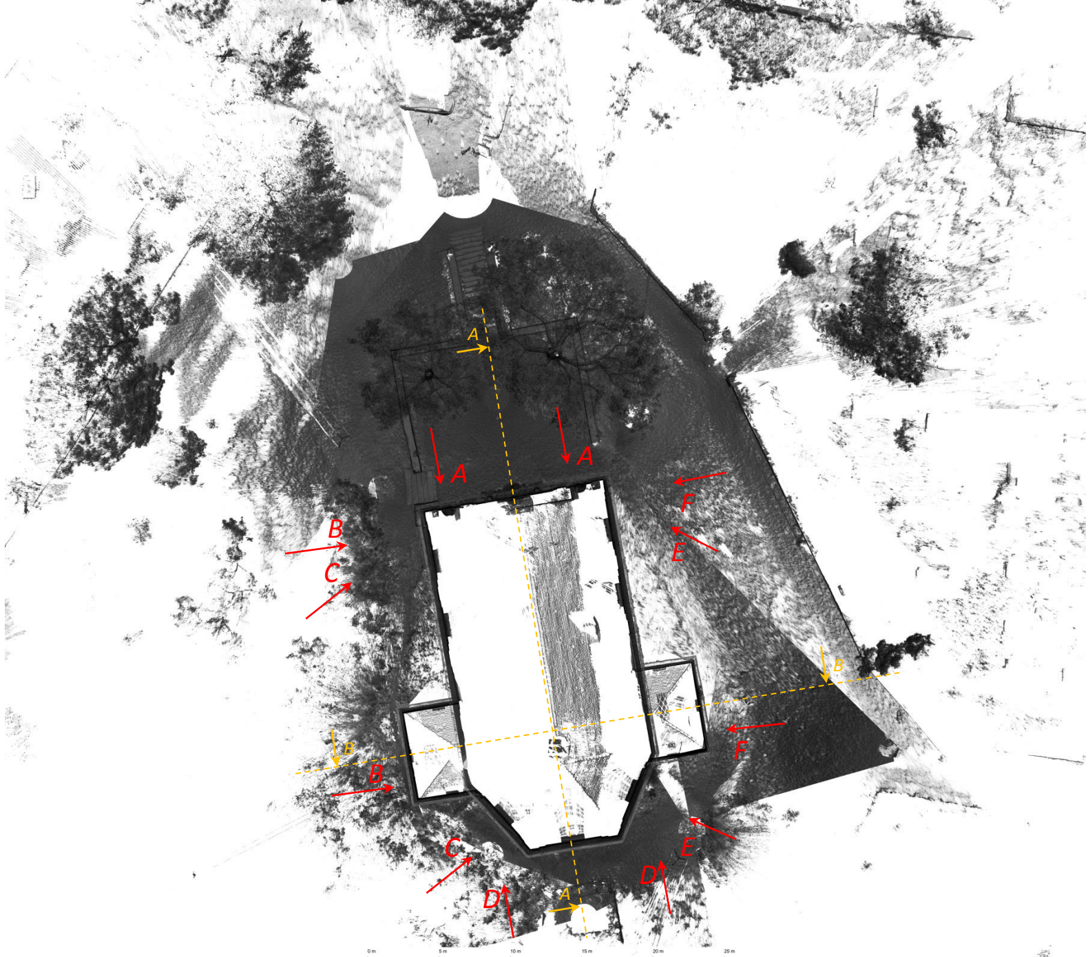
MÍLEŠOVICE - KOSTEL SV. ANTONÍNA PADUÁNSKÉHO - PŮDORYSNÝ POHLED
